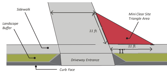
FIGURE 7.4.94 Mini Clear Sight Triangle
